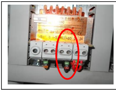
Figura 6 Trasformatore impostato a 460 V
