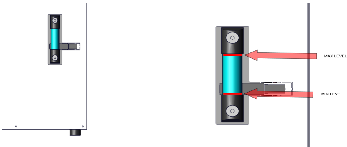
Figura 17 / 18 – Rabbocco del serbatoio
