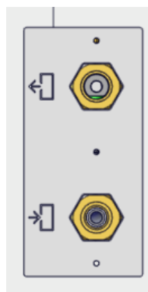
Figura 4 – Placa para las conexiones hidráulicas
