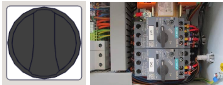
Abbildung 7 – Hauptschalter OFF Abbildung 8– Trennschalter OFF
