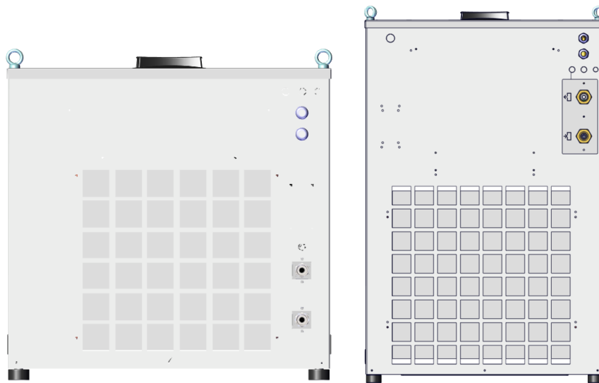
Рис. 20 – Внешняя поверхность конденсатора для CCE 6101 – 6201 – 6301
