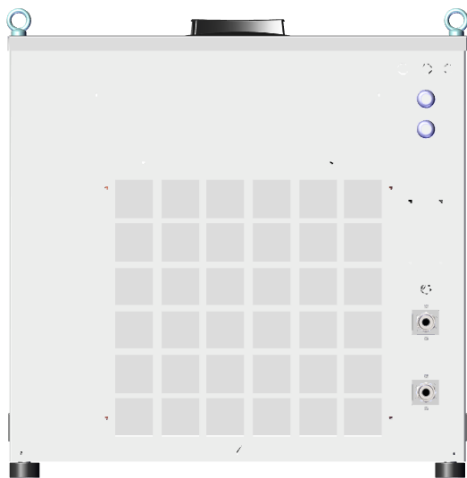
Picture 20 – Verflüssige Außenfläche für CCE 6101 – 6201 – 6301
