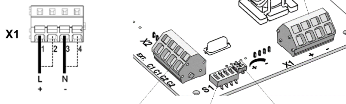
X2 Entrée de commande externe S1 Choix du mode opératoire Commande de l'intensité lumineuse (15 - 100 %)
