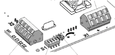
S1 Выбор режима работы Регулирование интенсивности освещения (15 – 100%)
