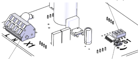
X1 Подключение рабочего напряжения Регулирование интенсивности освещения (15 – 100%)
